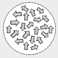
Броуновское движение
